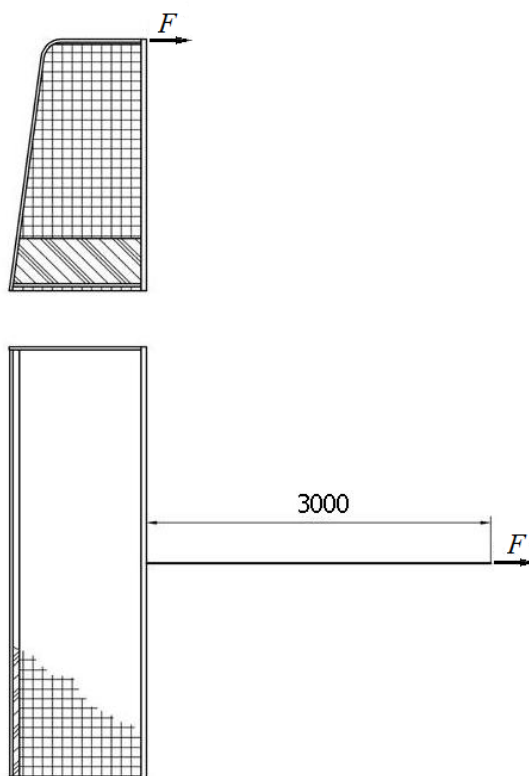
Рисунок Б.1 – Схема нагружения ворот
