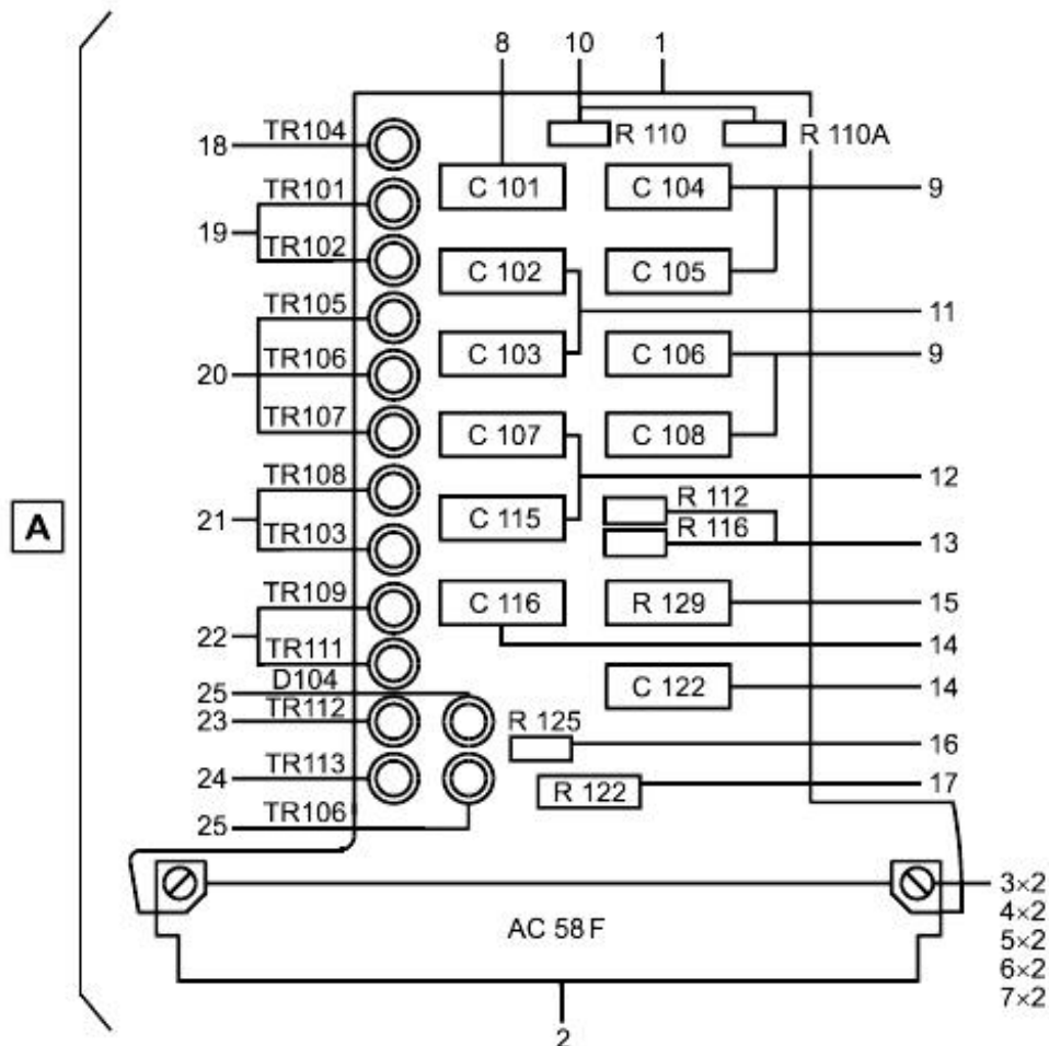
Рисунок В.3 - Пример идентификации электрических и электронных компонентов
